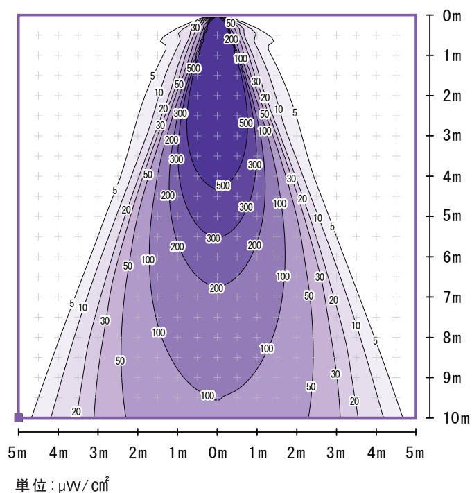
■ BL350-UV120-A6 (広角配光)
