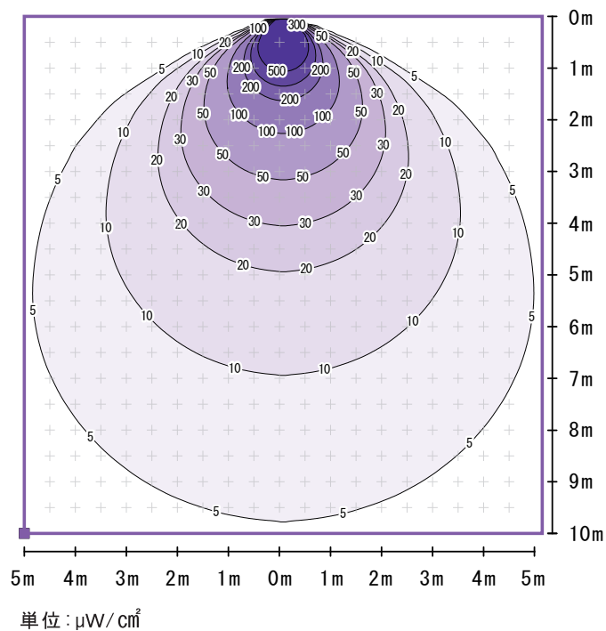
■ BL240-UV120 (広角配光)
