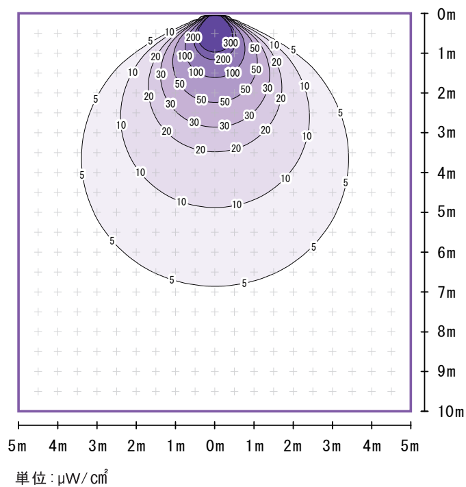
■ BL120-UV120-A6 (広角配光)
