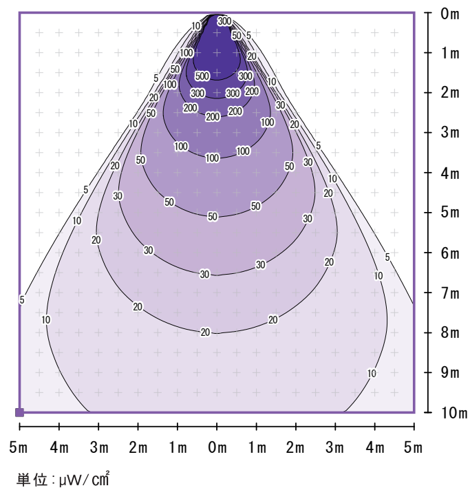
■ BL240-UV65 (広角配光)
