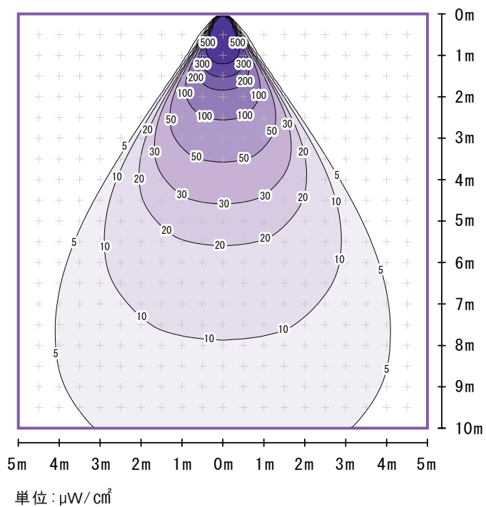
■ BL120-UV65-A6 (広角配光)
