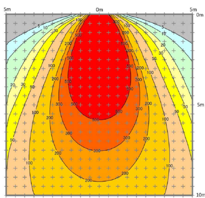
GL500C-WN40
