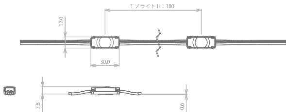
製品外形図
