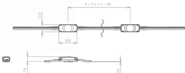
製品外形図
