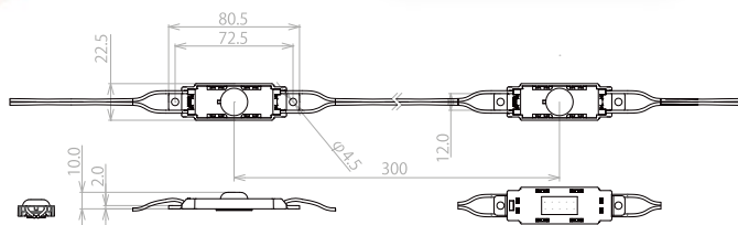
製品外形図
