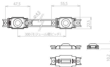
製品外形図
